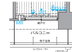
◇ C3TYPE 213号室部分図
