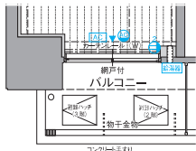
◇ D1TYPE 2・3階部分図
