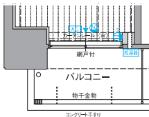
◇ A1TYPE 2階部分図
