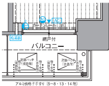
◇ A2TYPE 5~15階部分図
