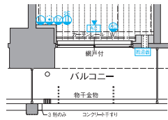
◇ C2TYPE 304・306・406号室部分図
