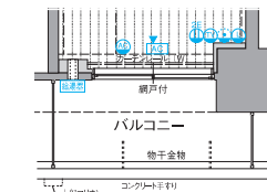
◇ C3TYPE 211号室部分図
