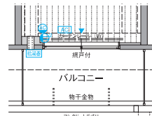
◇ B3TYPE 2階部分図
