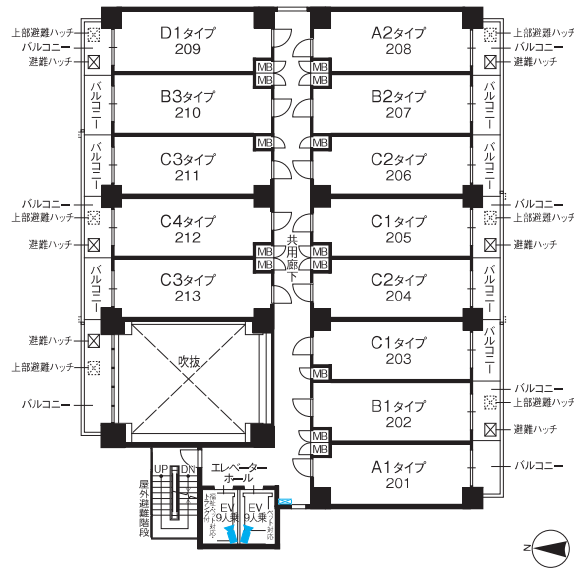
◇ 2階平面図 scale 約1/350
