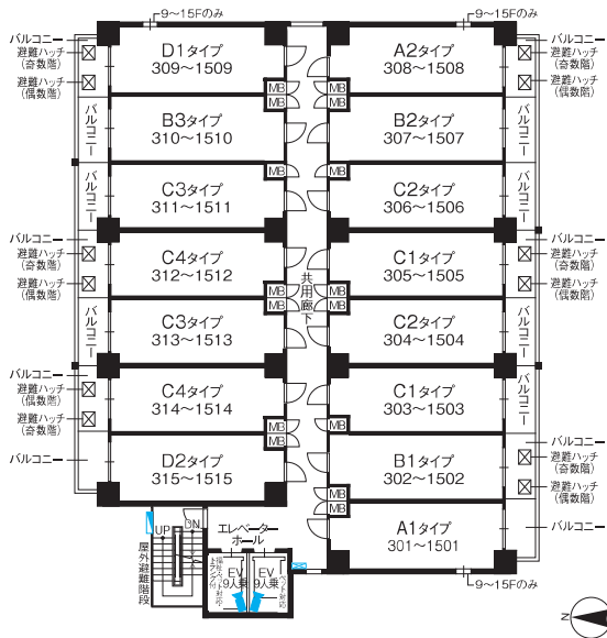
◇ 3～15階平面図 scale 約1/350
