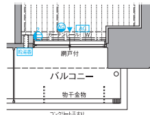
◇ D2TYPE 3階部分図
