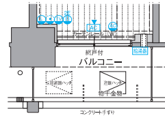
◇ C4TYPE 314号室部分図
