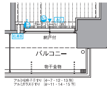
◇ D2TYPE 4~15階部分図
