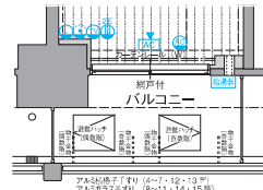
◇ C4TYPE 414~1514号室部分図
