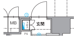
◇ C3TYPE 213~1513号室部分図
